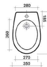
Bidet a terra
