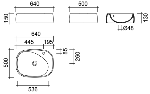
Lavabo da appoggio H150 28LVB
