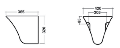
Lavabo sospeso 24 LV Colonna sospesa 24CLS
