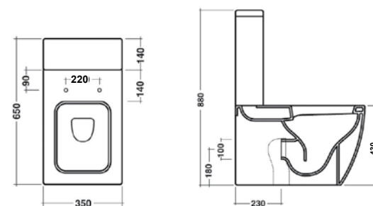
Vaso monoblocco + cassetta 22MBS/P + 22CM
