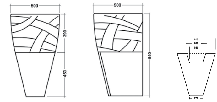
Lavabo sospeso H390 22LV
