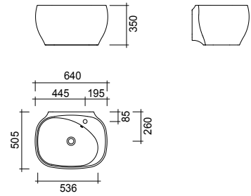
Lavabo sospeso 28LV
