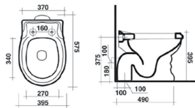
Vaso a terra/parete 13VS/P
