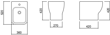
Bidet a terra
