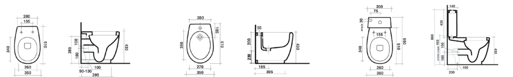
Vaso a terra 29VS/P Bidet a terra 29BDM Vaso monoblocco + cassetta 29MBS/P + 29CM
