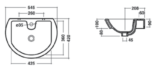
Lavabo sospeso 24 LV Colonna sospesa 24CLS
