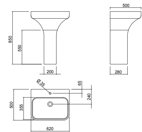
Lavabo + colonna
