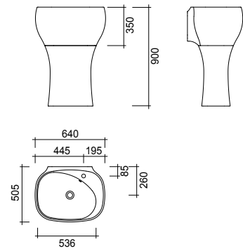
Lavabo + colonna a righe 28LV+28CLR
