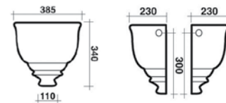
Cassetta alta 13CA
