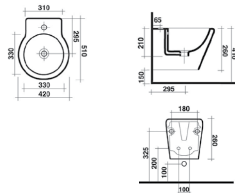
Bidet sospeso 16BDS
