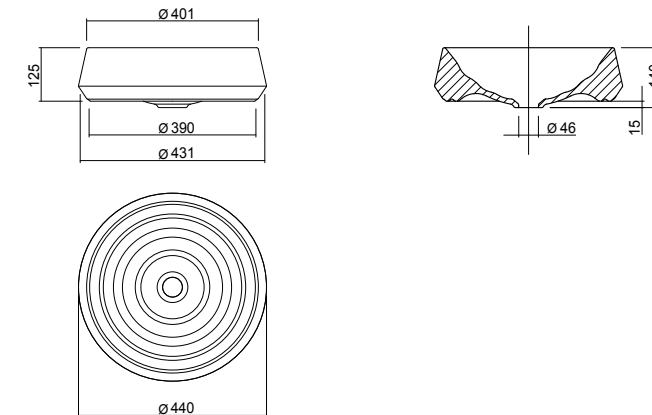
Lavabo da appoggio UP
