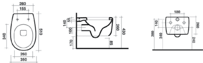
Vaso sospeso
