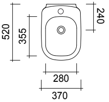
Bidet sospeso
