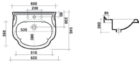
Lavabo semincasso 13LI
