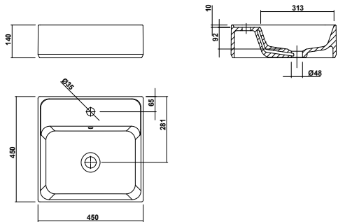
Lavabo da appoggio KLASS 45 KLA45 Lavabo da appoggio KLASS 60 KLA60
