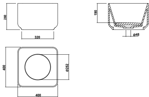
Lavabo da appoggio SPEED 40 SPE401 Lavabo da appoggio SPEED S40 SPE402
