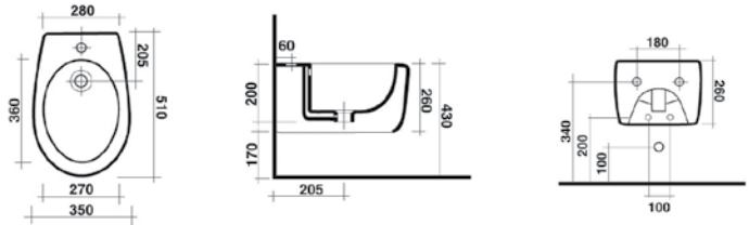
Bidet sospeso
