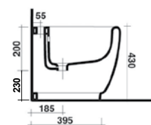
Bidet a terra
