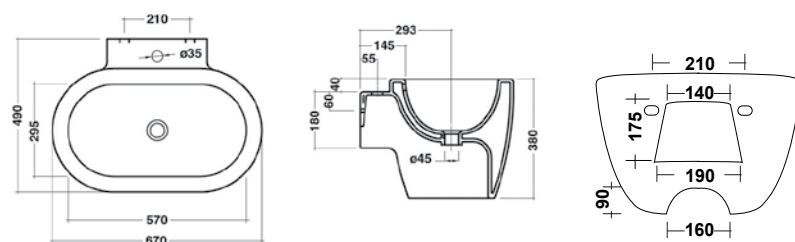
Lavabo sospeso 23LV
