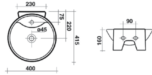
Lavabo da appoggio e sospeso TWIN TW304
