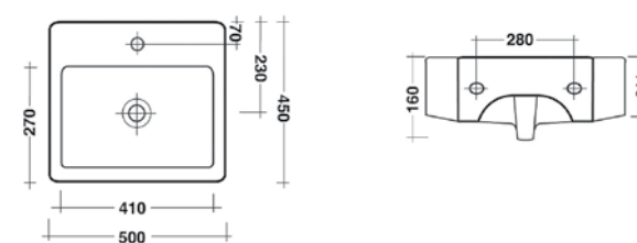
Lavabo da appoggio
