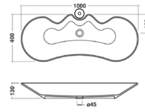
Lavabo da appoggio FLY DOPPIO F316 Porta rubinetto ceramica PR01
