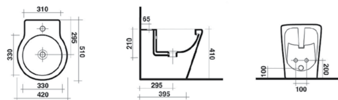
Vaso a terra 16VS/P Bidet a terra 16BDM
