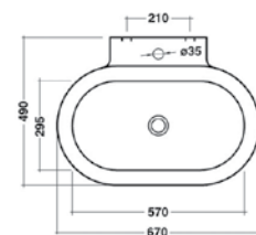
Lavabo sospeso 27LV
