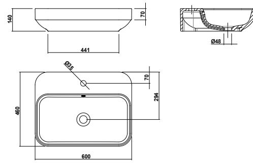
Lavabo da appoggio SPACE 50 SPA50 Lavabo da appoggio SPACE 60 SPA60
