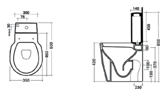
Vaso monoblocco + cassetta 24MBS/P + 24CM
