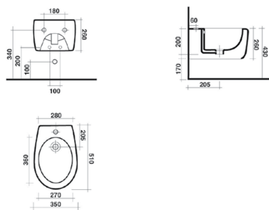
Bidet sospeso
