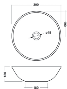
Lavabo da appoggio WORD
