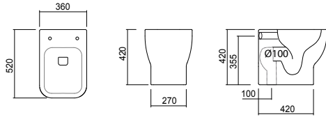
Vaso a terra
