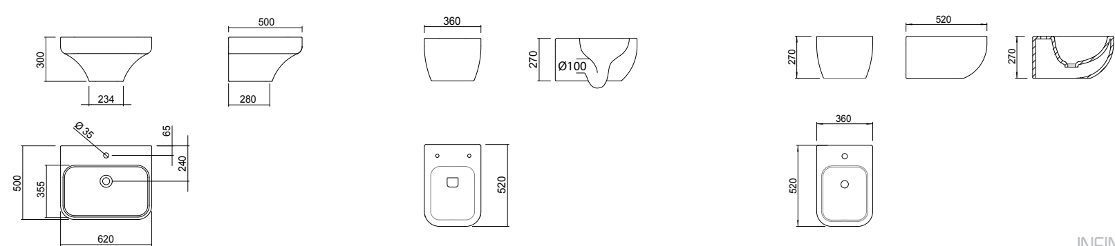
Lavabo sospeso 30LV Vaso sospeso 30VSO Bidet sospeso 30BDS
