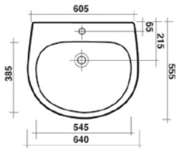
Lavabo sospeso
