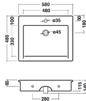
Lavabo da appoggio, incasso, sospeso WISH W313
