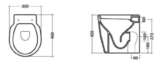
Vaso a terra 24VS/P
