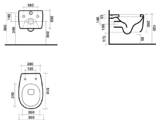
Bidet sospeso
