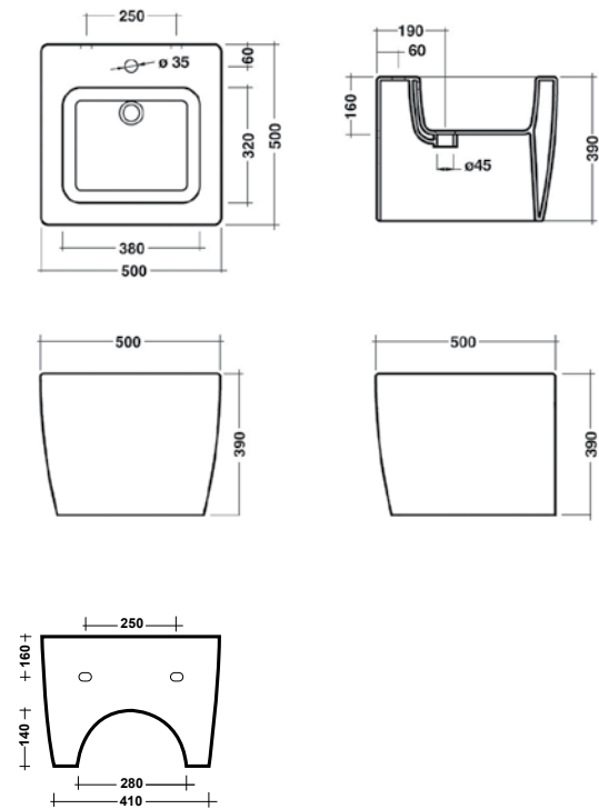
Lavabo + mobile 26LV + 26MBL
