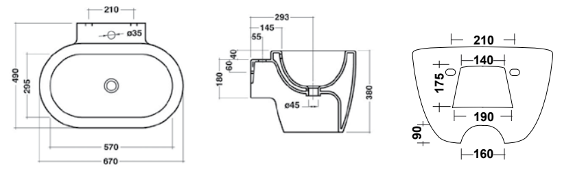
Lavabo sospeso 29LV
