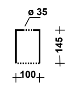
Lavabo da appoggio FLY SINGOLO F317 Porta rubinetto ceramica PR01
