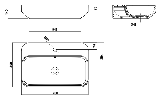
Lavabo da appoggio SPACE 70 SPA70
