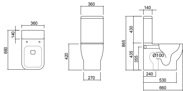
Vaso monoblocco + cassetta 30MBS/P + 30CM
