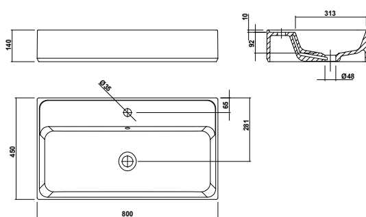
Lavabo da appoggio KLASS 80 KLA80 Lavabo da appoggio KLASS 100 KLA100
