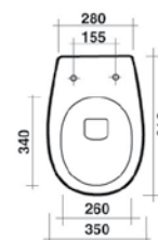
Vaso a terra
