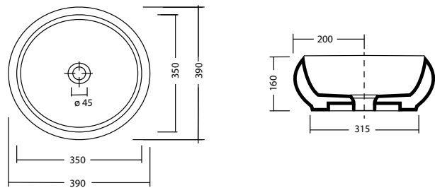
Lavabo da appoggio SOFT
