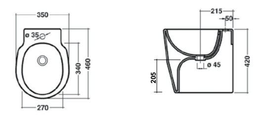
Bidet a terra 24BDM
